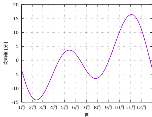
図 2: 均時差
